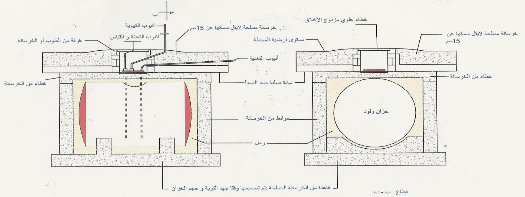
شكل (2) يوضح خزان الوقود داخل حوض من الخرسانة
