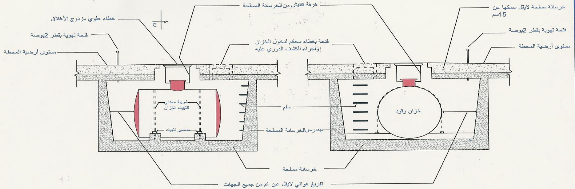
شكل (1) يوضح خزان وقود داخل غرفة من الخرسانة
