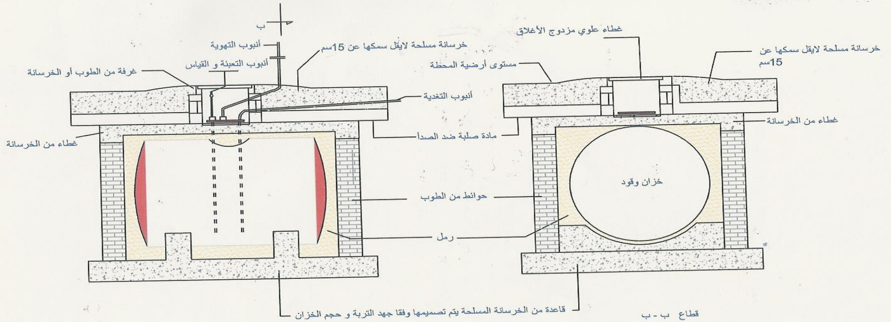
شكل (3) يوضح خزان الوقود داخل حوض من الطوب
